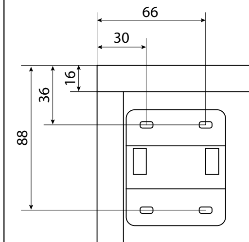
Схема присадки
