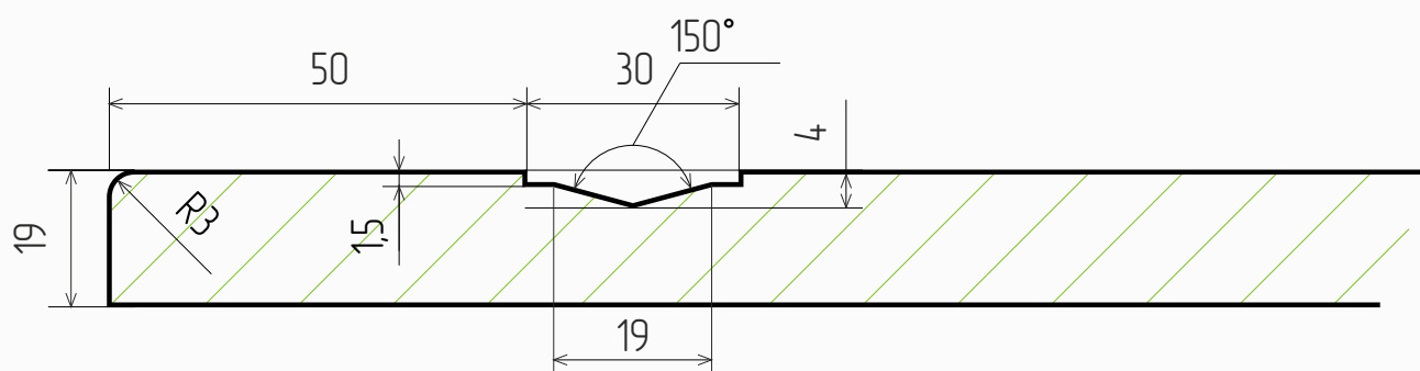
Глухой фасад
