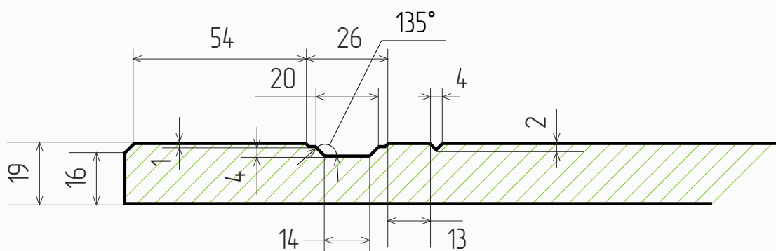
Глухой фасад
