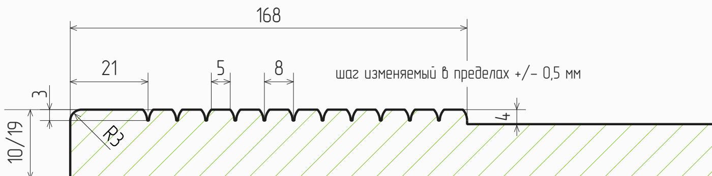
Глухой фасад
